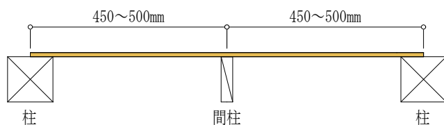
図 20 1P 耐力壁 納まり図
