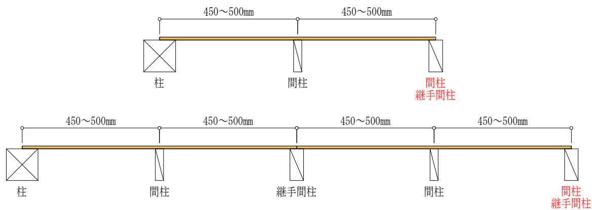
図 25 端部が間柱および継手間柱の壁 納まり図
